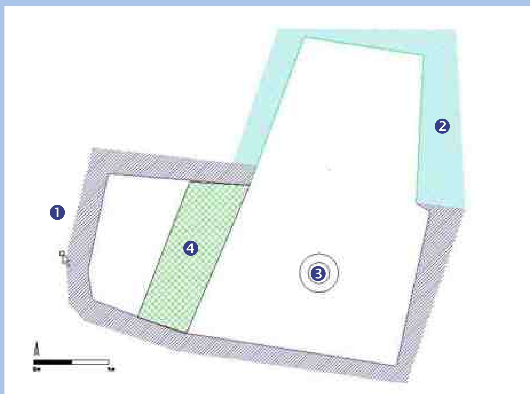
Grundriss des Gefängnisses
